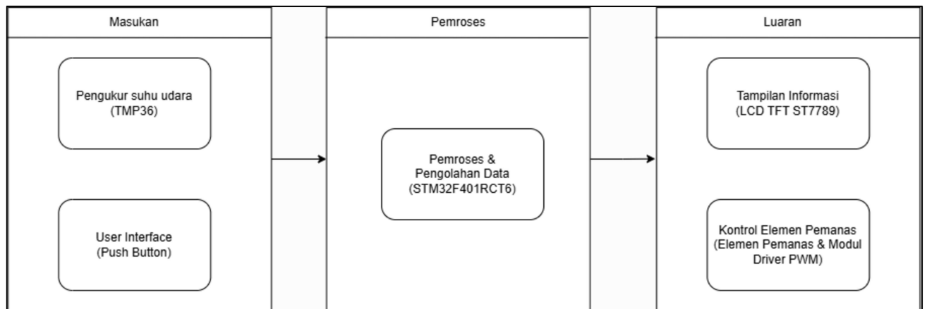
Diagram Blok Sistem Modul Pemanas Udara
